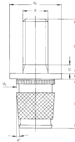
Type 0941 ④
